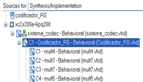
Fig. 3 Jerarquía de componentes del codificador.
