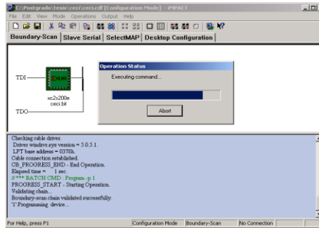
Fig. 7 Proceso de programación del FPGA.
