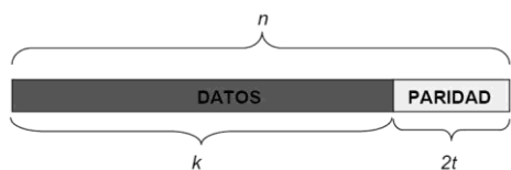
Fig. 1 Palabra de código Reed- Solomon (Clemente, 2004).
