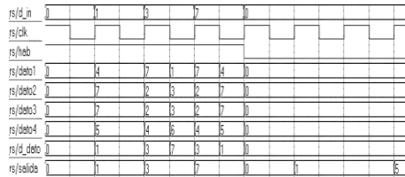
Fig. 8 Simulación del codificador RS.
